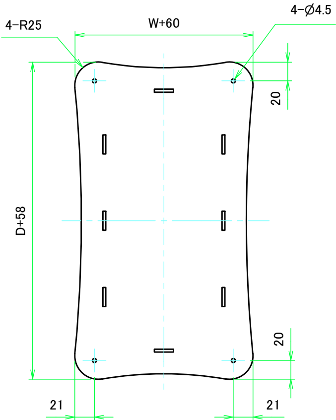
上カバー表面 / Top cover Frontside
