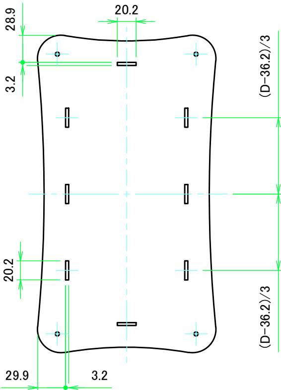
上カバー裏面 / Top cover Backside
