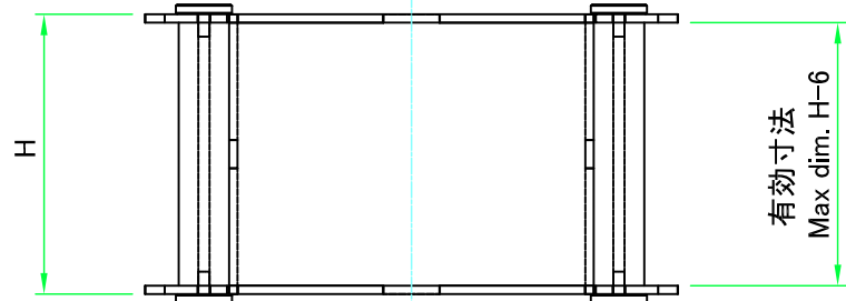
Wパネル1 / W panel 1
